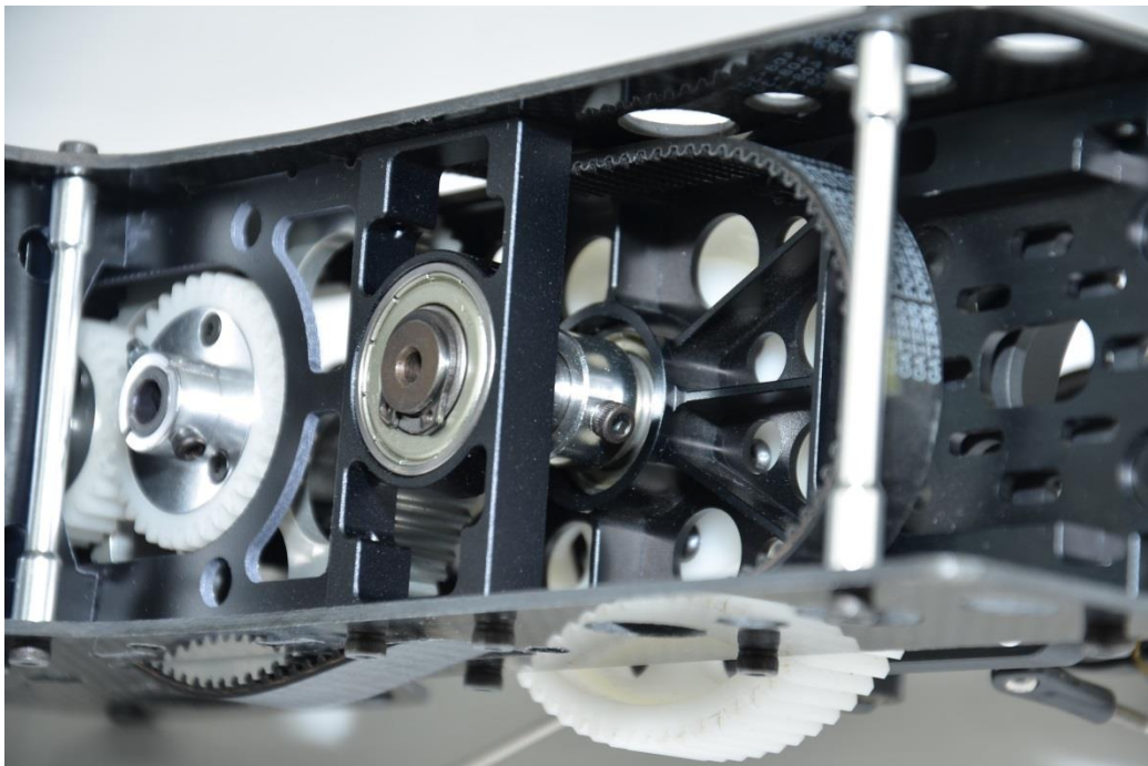
3-fach gelagerte Hauptrotorwelle geänderte Sicherung
