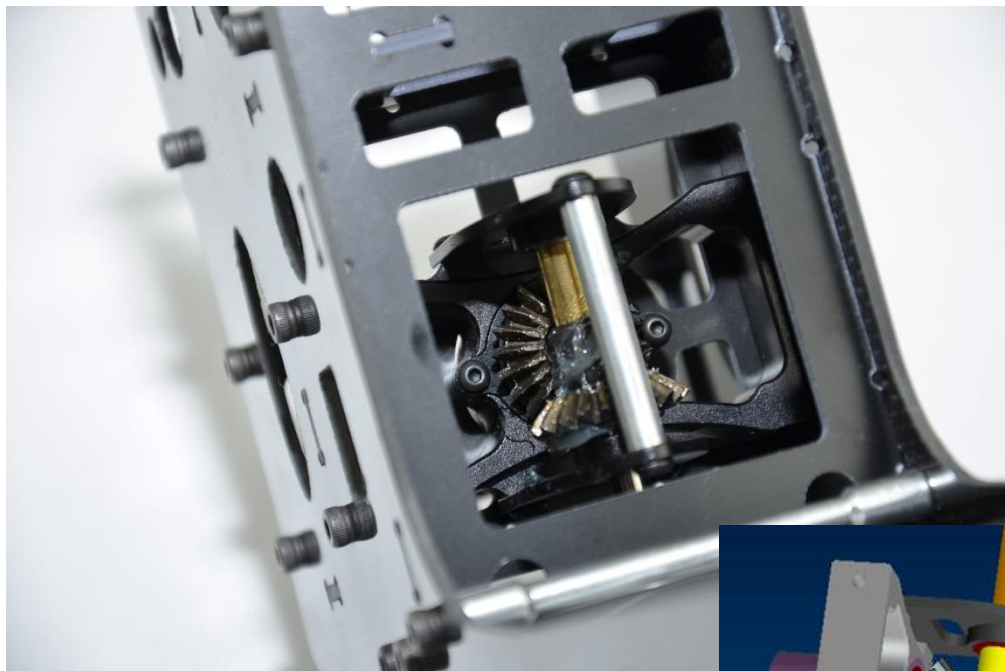
Komplett geänderter Heckabtrieb
